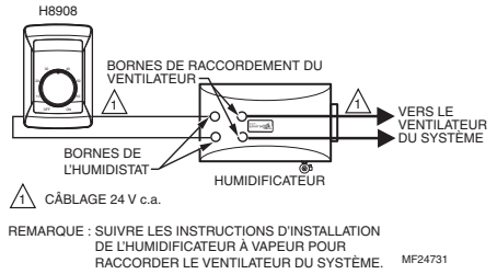
Fig. 16. Raccordement du H8908 avec un humidificateur à vapeur.
