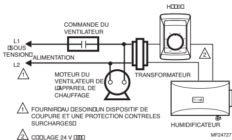
Fig. 12. Raccordement du H8908 avec asservissement du ventilateur.
