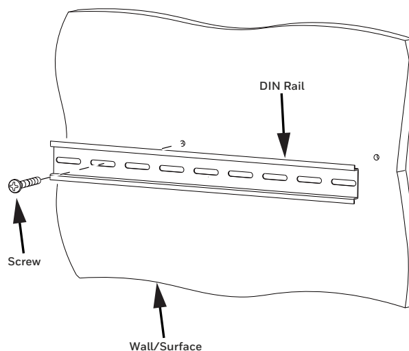
Fig. 6 DIN Rail Wall/Surface
