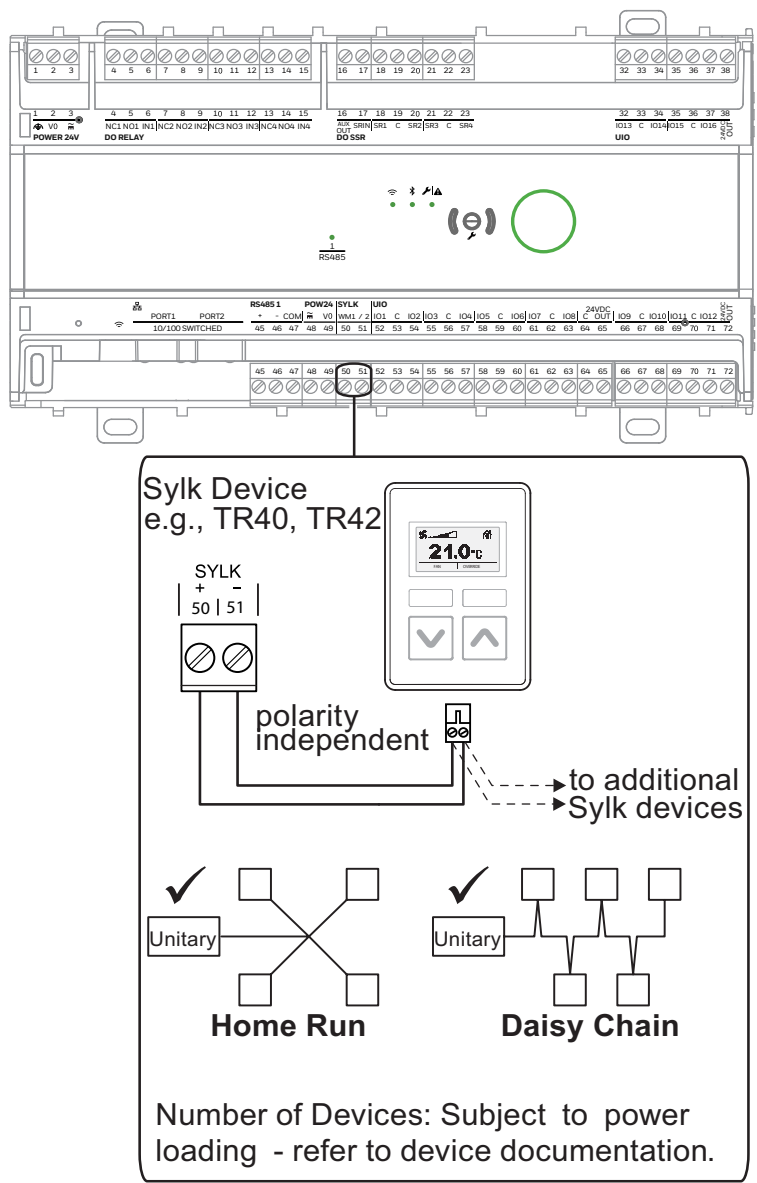
Fig. 31 Sylk™ Wiring Topologies
