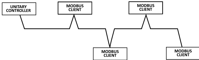
Fig. 29 Modbus Wiring Topology
