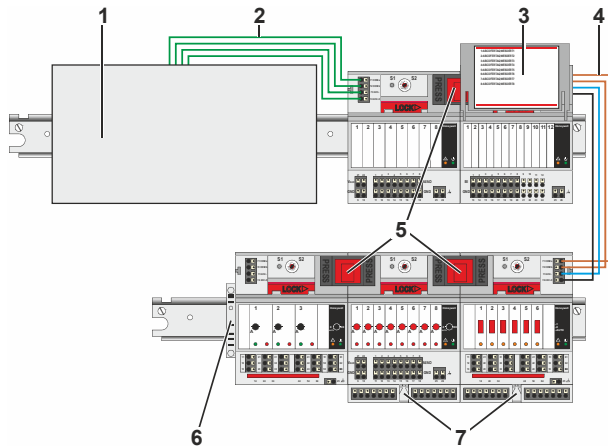
Fig. 2. Panel Bus I/O Modules on DIN rails
